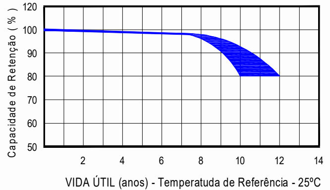
VIDA ÚTIL EM FLUTUAÇÃO - MODELOS DE 33 a 250 Ah
